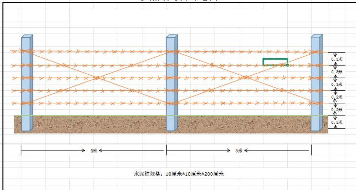
机械围栏安装示意图
