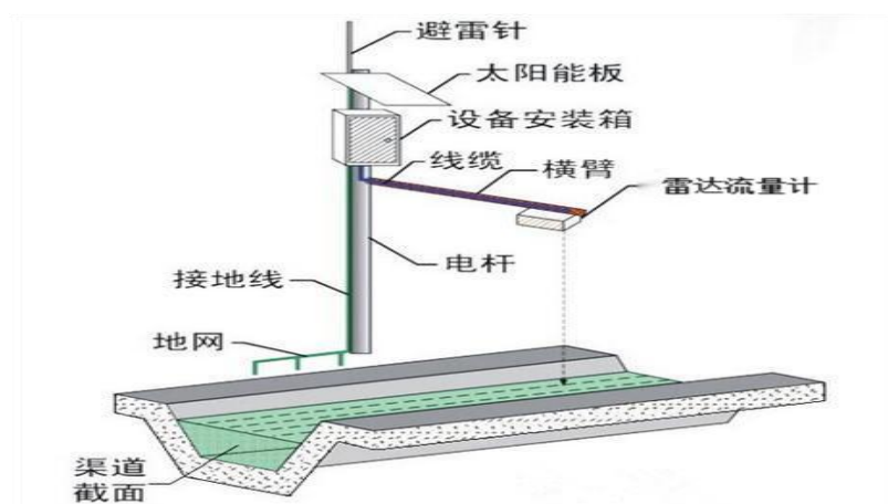
图 3 雷达流量计安装示意图
