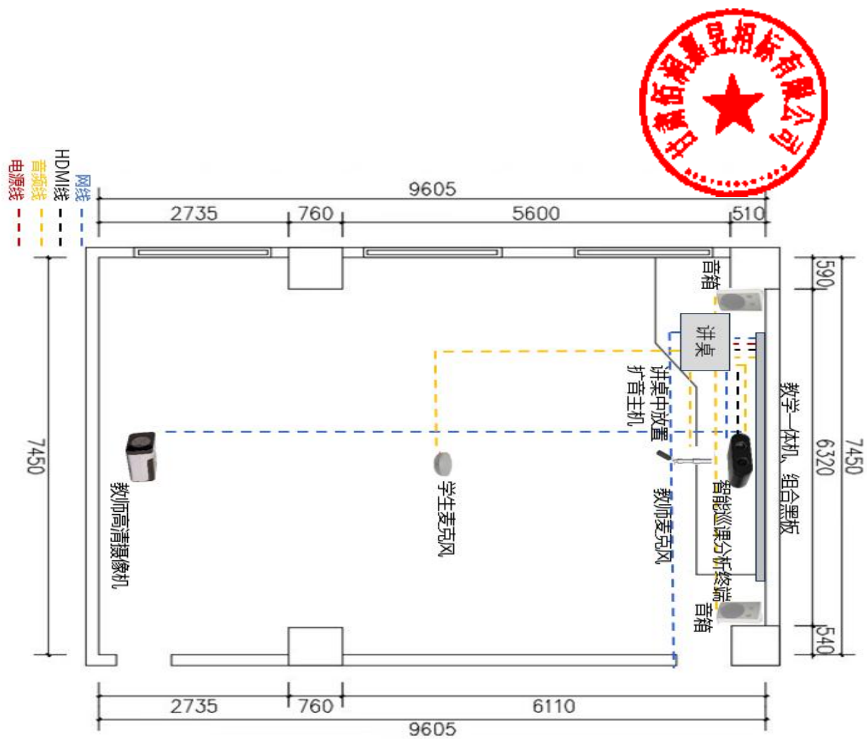
图 2：二号教学楼 61 间智慧教室布线图
