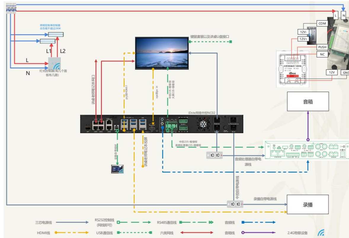
图 10：网络中控连线图
