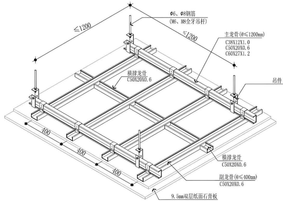
图 12：四号教学楼 76 间教室吊顶示意图
