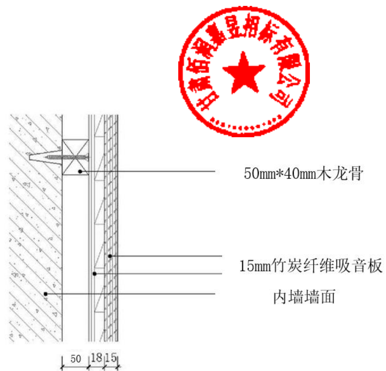
图 13：四号教学楼 35 间教室前墙吸音处理示意图
