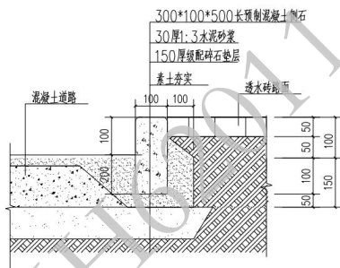
路缘石做法详图 1:25
