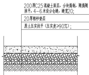
场地硬化断面图 1:25
