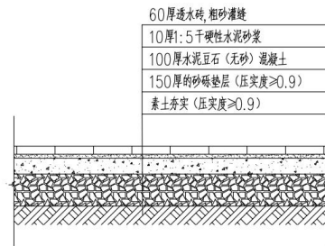
透水砖铺装做法 1:25
