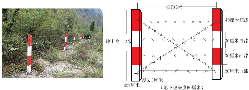
图 1 围栏示意图
