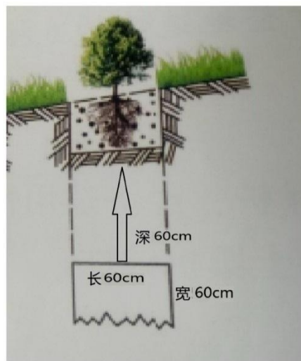
方形穴状整地剖面图
