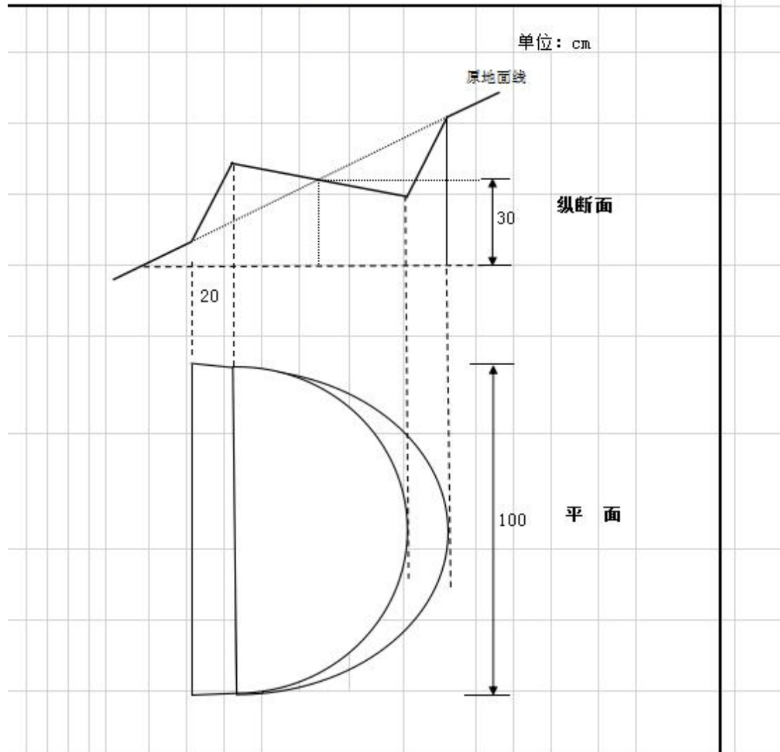
反坡鱼鳞坑整地纵断面、平面图
