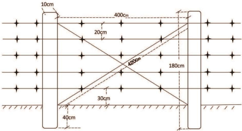
机械围栏示意图
