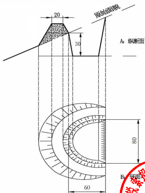
鱼鳞坑整地示意图
