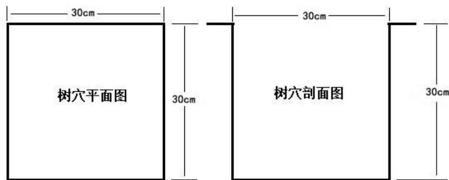
图 2-2 灌木定植穴配置图
