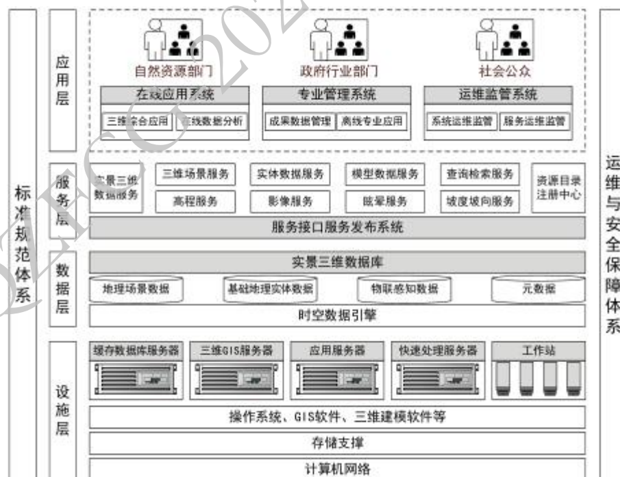
图 1 酒泉市实景三维数据库系统架构
