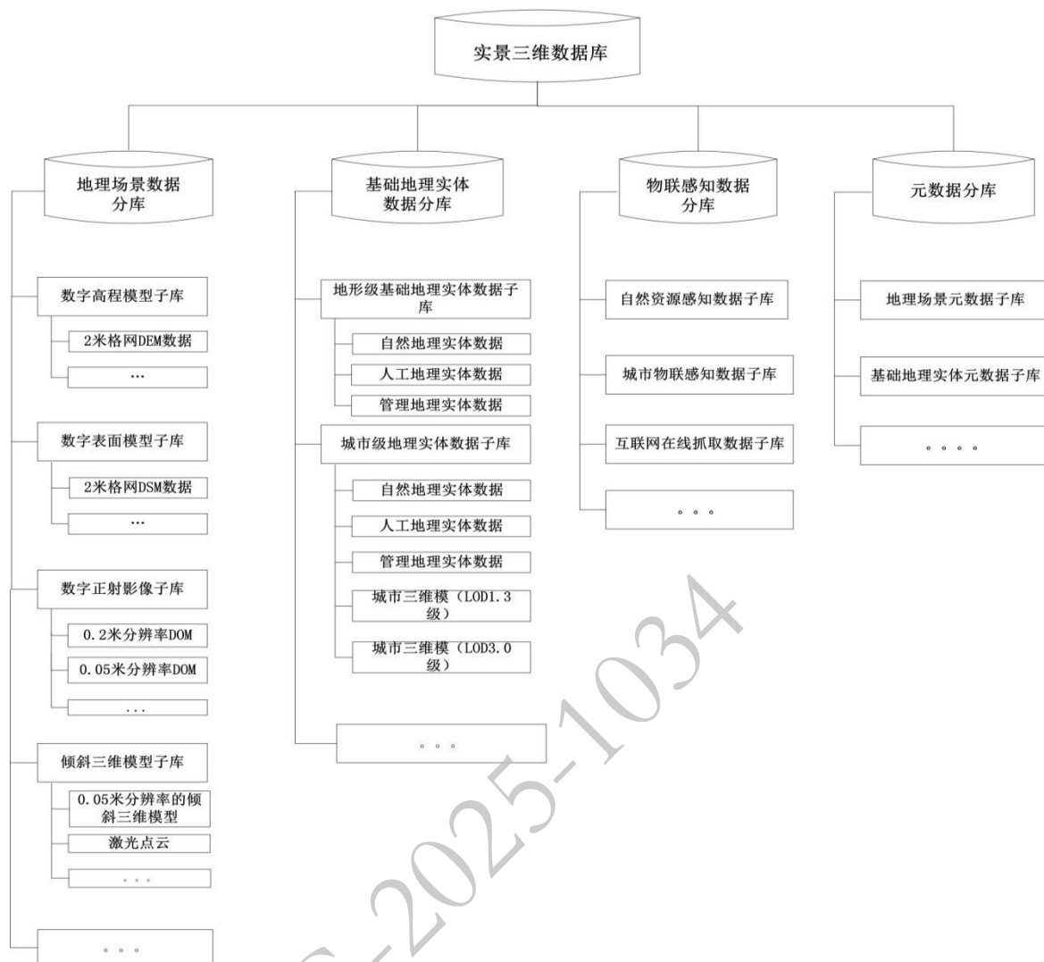
图 2 实景三维数据库总体结构
