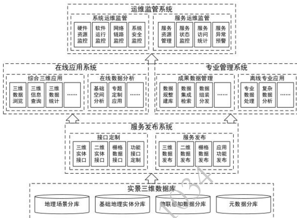
图 3 数据库管理系统功能模块
